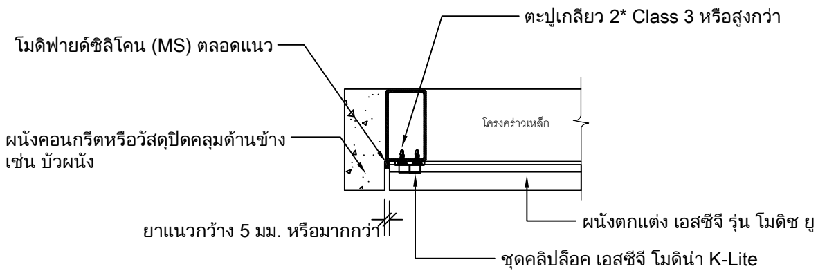
Detail ผนังคอนกรีตหรือวัสดุปิดคลุมด้านข้าง กรณีชนขอบคอนกรีต
