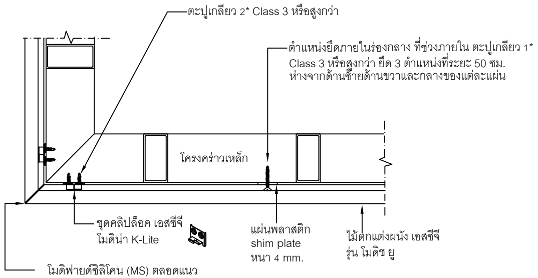
Detail ใช้งานบริเวณภายนอก
