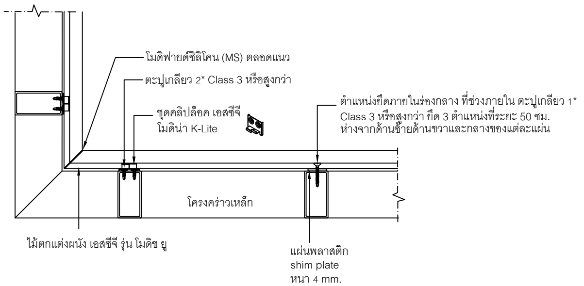
Detail ใช้งานบริเวณมุมใน
