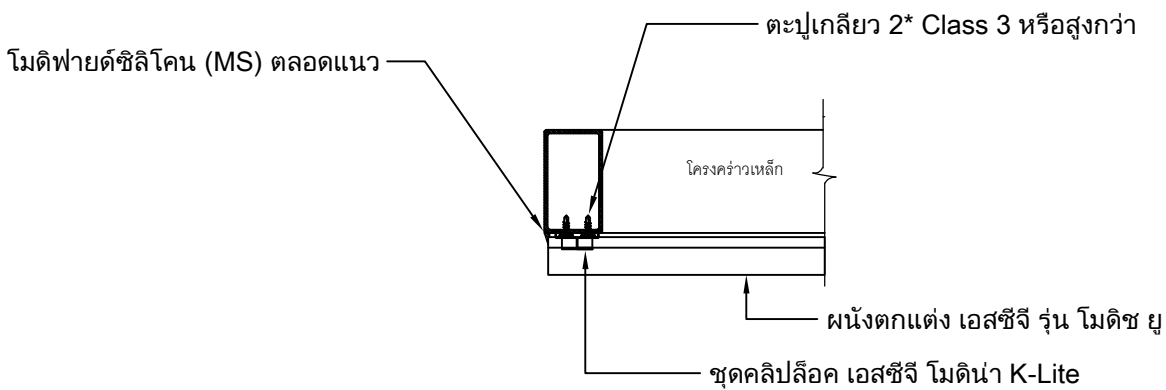
Detail ผนังคอนกรีตหรือวัสดุปิดคลุมด้านข้าง กรณีไม่ชนขอบคอนกรีต
