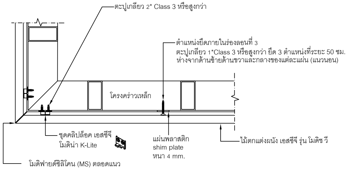
Detail จบงานบริเวณภายนอก
