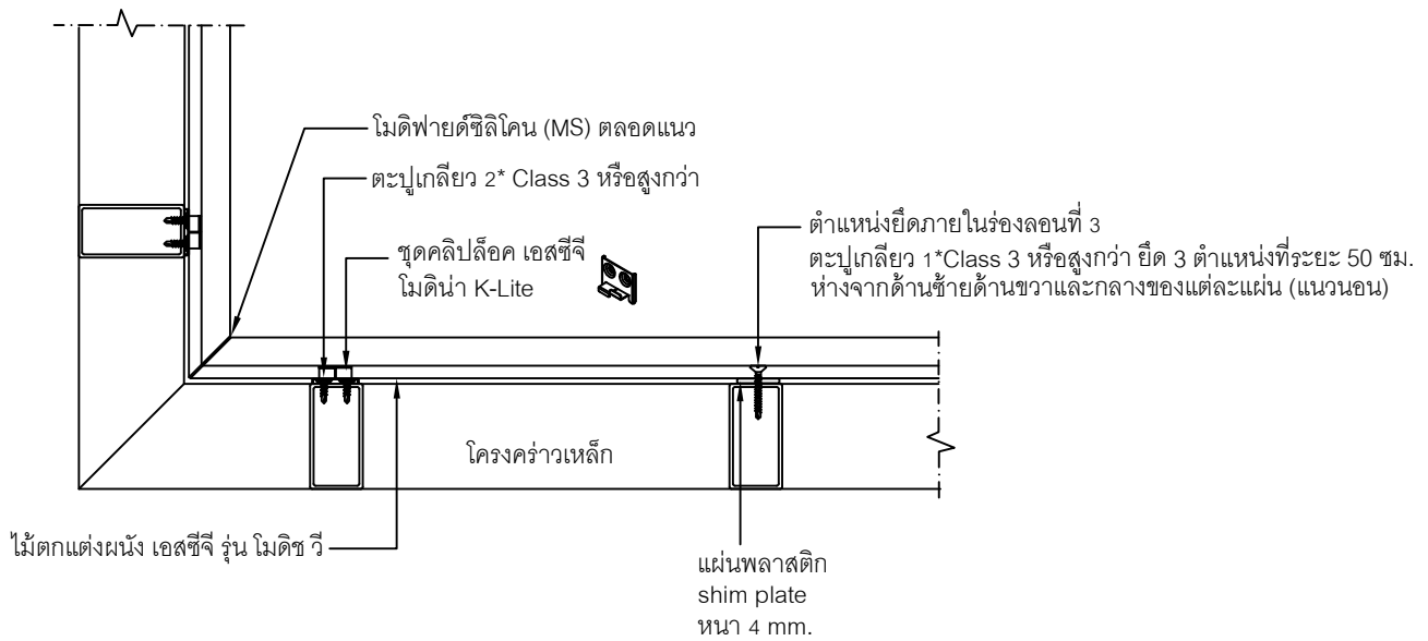
Detail จบงานบริเวณมุมใน
