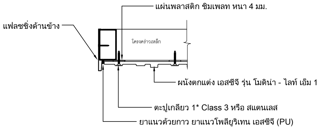
Detail ผนังด้านข้าง กรณีไม่ชนขอบคอนกรีต
