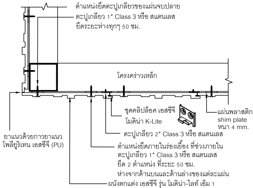
Detail จบงานมูนอก
