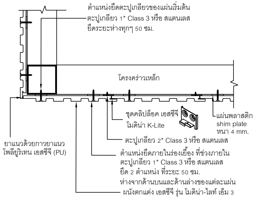
Detail งานมุนนอก
