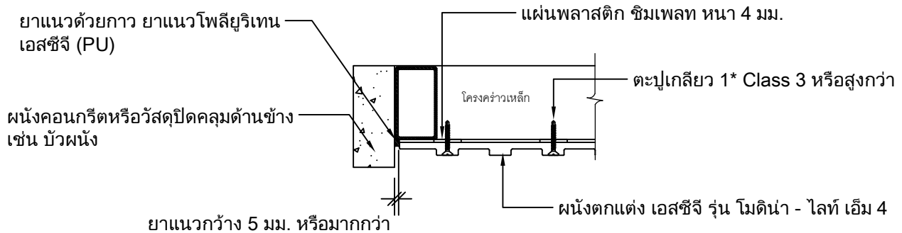
Detail จบงานด้านข้าง กรณีชนขอบคอนกรีต
