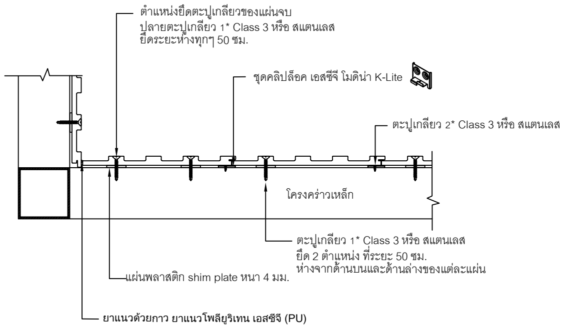
Detail จบงานบริเวณมุมใน
