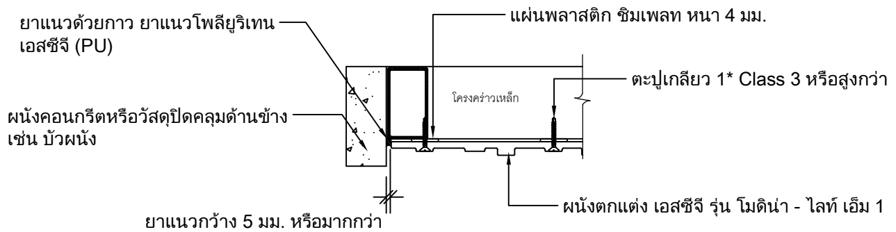
Detail ผนังด้านข้าง กรณีชนขอบคอนกรีต
