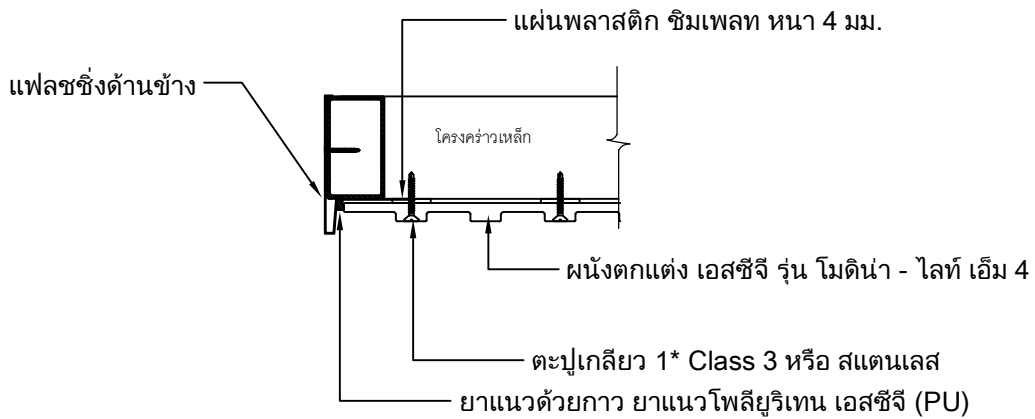
Detail จบงานด้านข้าง กรณีไม่ชนขอบคอนกรีต
