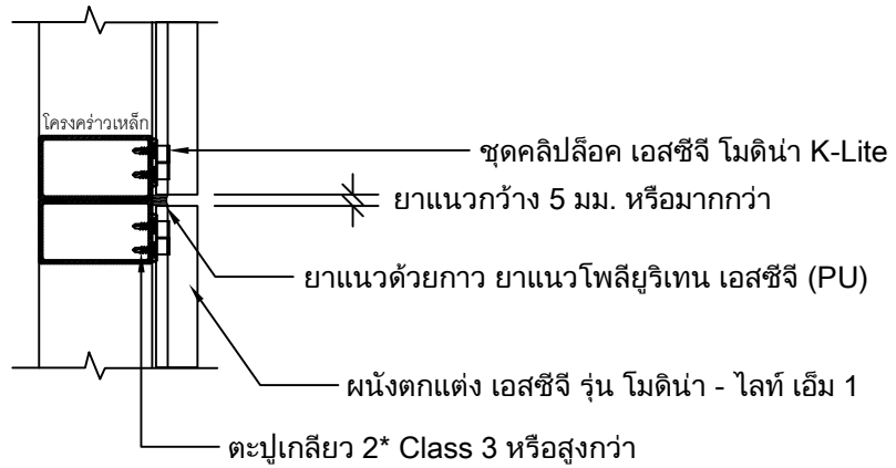
Detail รอยต่อระหว่างแผ่น
