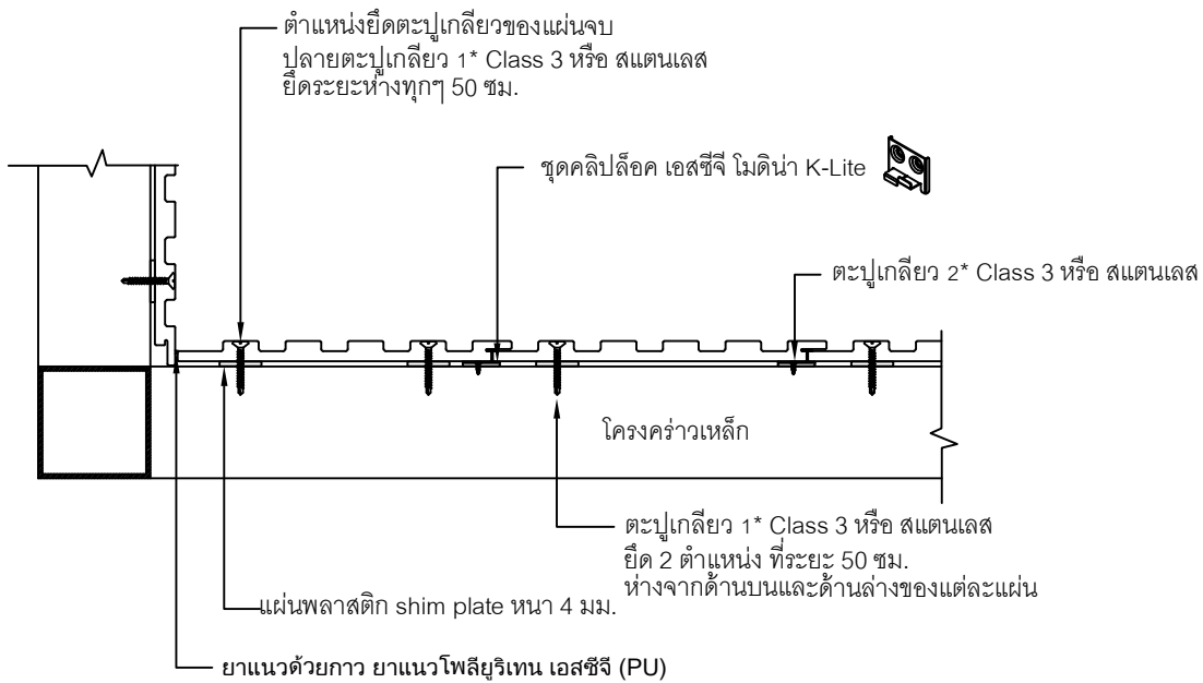
Detail งานบริเวณมุมใน
