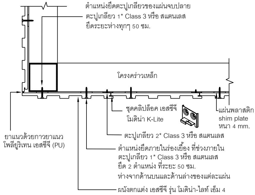
Detail จบงานมุมนอก
