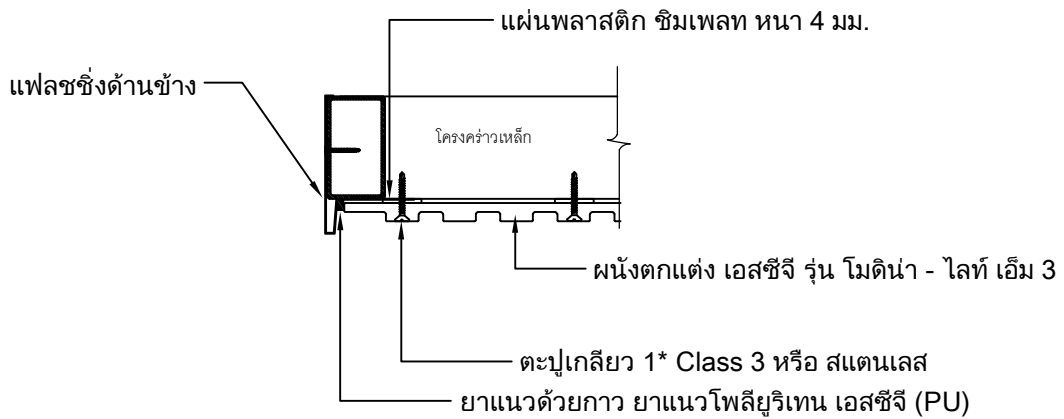
Detail จบงานด้านข้าง กรณีไม่ชนขอบคอนกรีต
