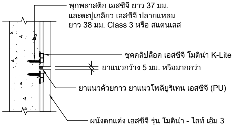
Detail รอยต่อระหว่างเฟรม
