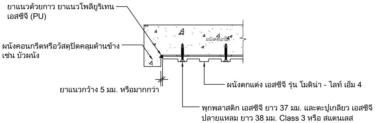
Detail จบงานด้านข้าง กรณีชนขอบคอนกรีต
