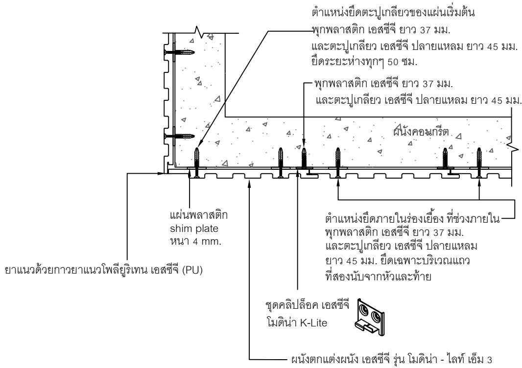
Detail ภายนอก
