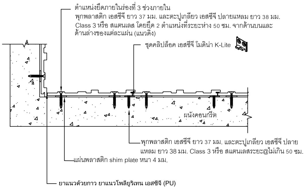
Detail ใช้งานบริเวณมุมใน
