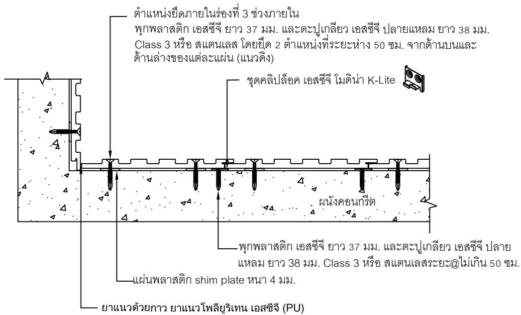
Detail บริเวณมุมใน
