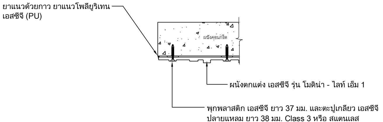
Detail จบงานด้านข้าง กรณีไม่ชนขอบคอนกรีต
