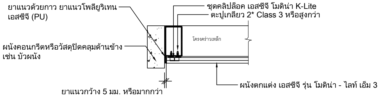
Detail ใช้งานด้านข้าง กรณีชนขอบคอนกรีต
