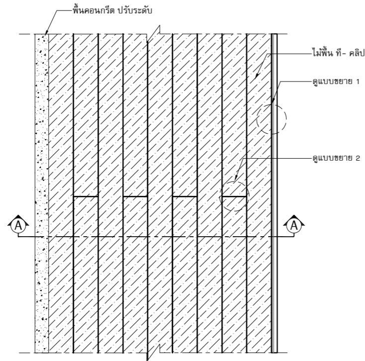
แปลน (ไม่น้ำ T-clip ชิลด์)
