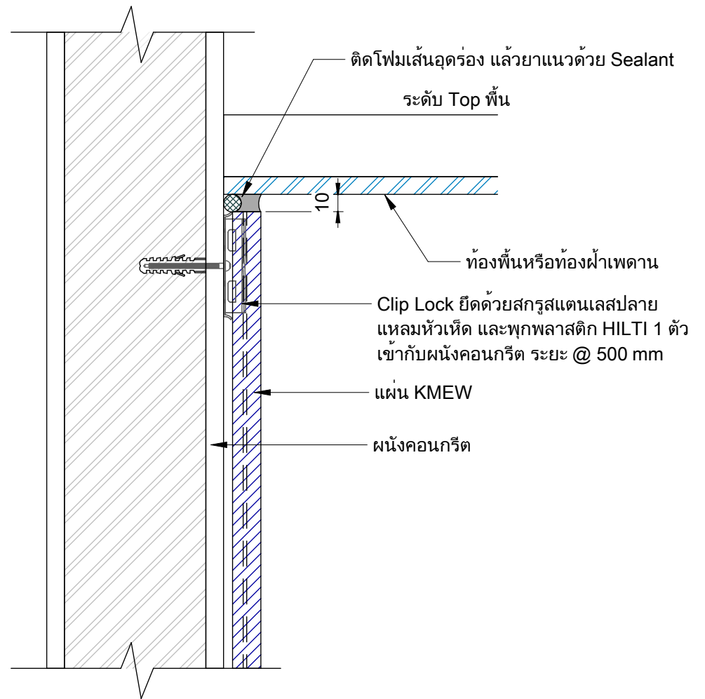
Section Detail - กรณีแผ่น KMEW ใช้งานด้วย Sealant
