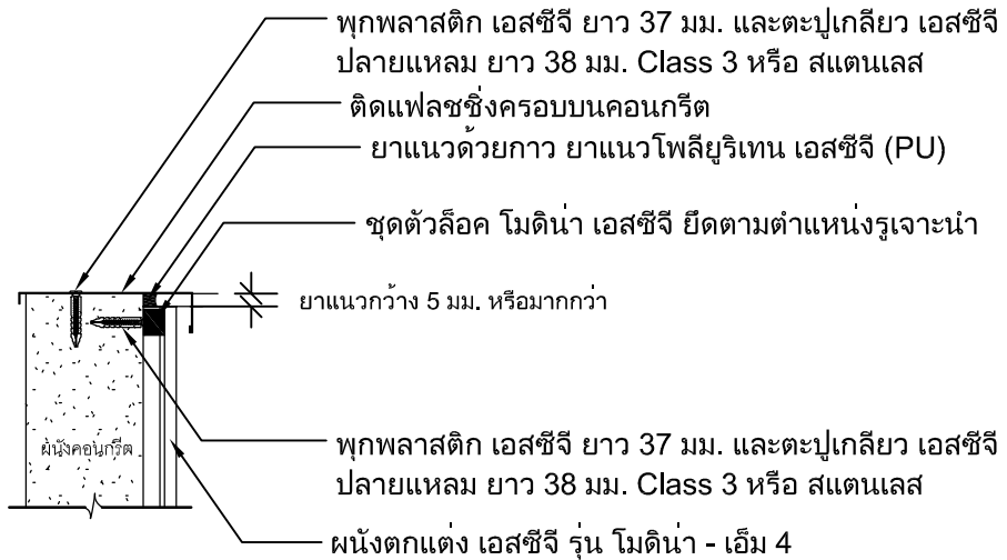
Detail ๒ งานด้านบน (กรณีผนังภายนอก)
