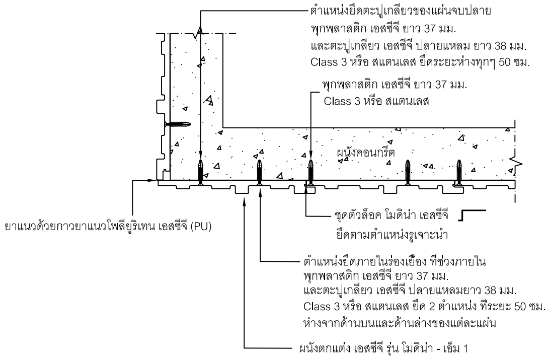
Detail ใช้งานมุมนอก
