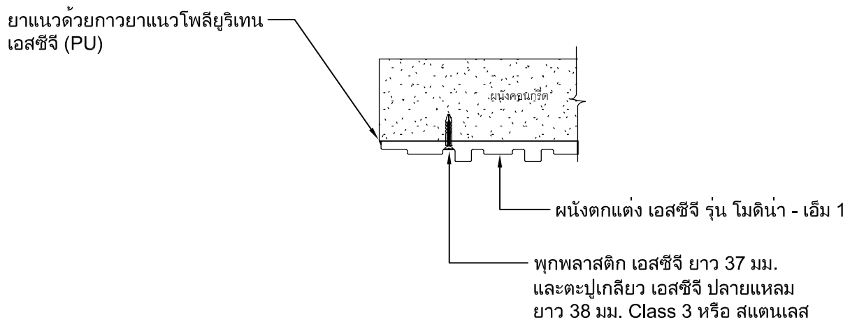
Detail ใช้งานด้านข้าง กรณีไม่ชนขอบคอนกรีต
