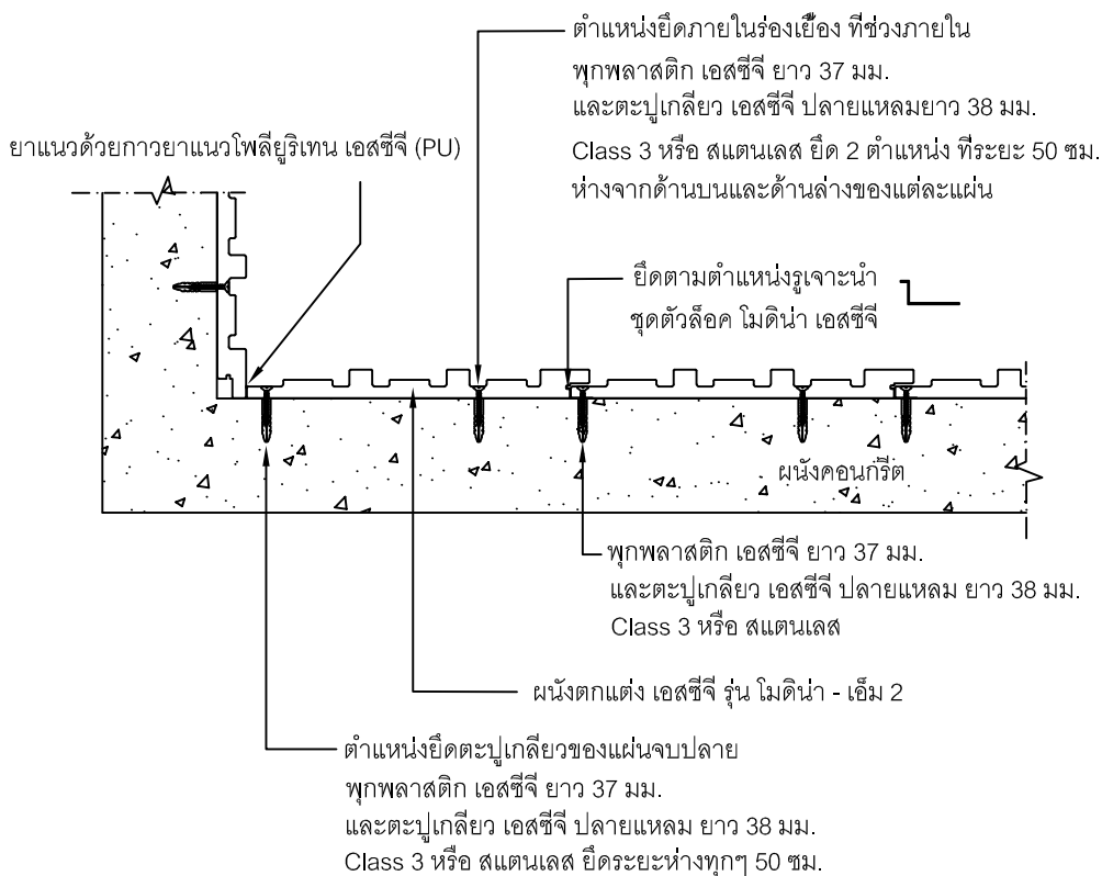
Detail จบงานมูนใน
