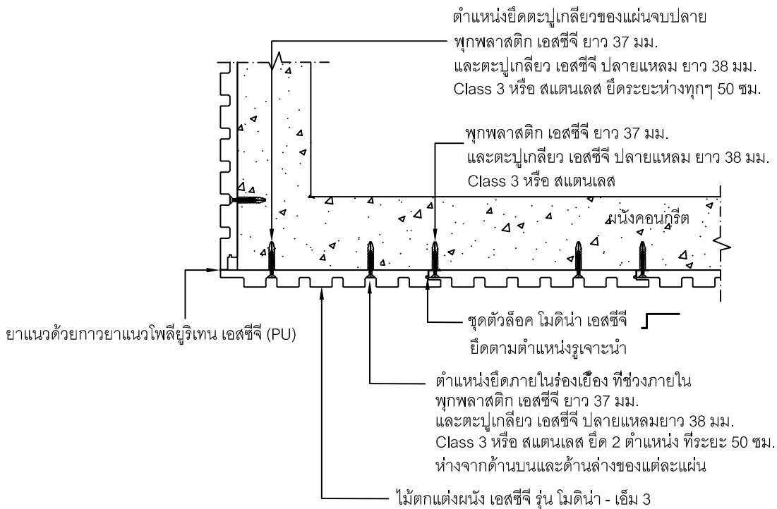
Detail ใช้งานมุมนอก
