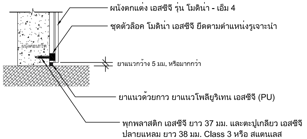
Detail ๓ งานด้านล่าง (กรณีเริ่มบนคอนกรีต)
