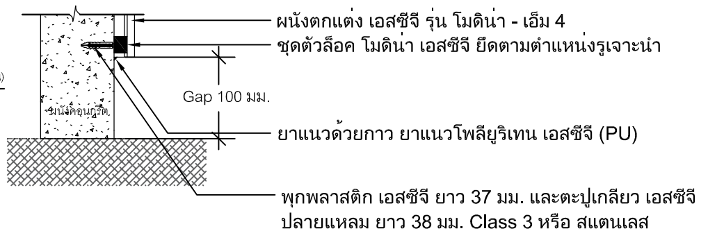
Detail ๔ งานด้านล่าง (กรณีเริ่มบนหินดิน)
