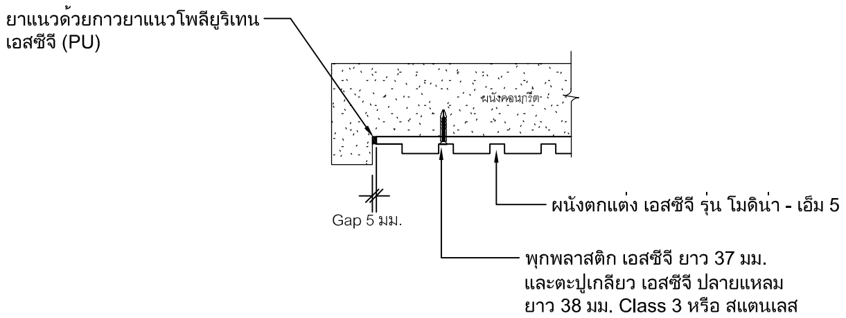
Detail จบงานด้านข้าง กรณีชนขอบคอนกรีต
