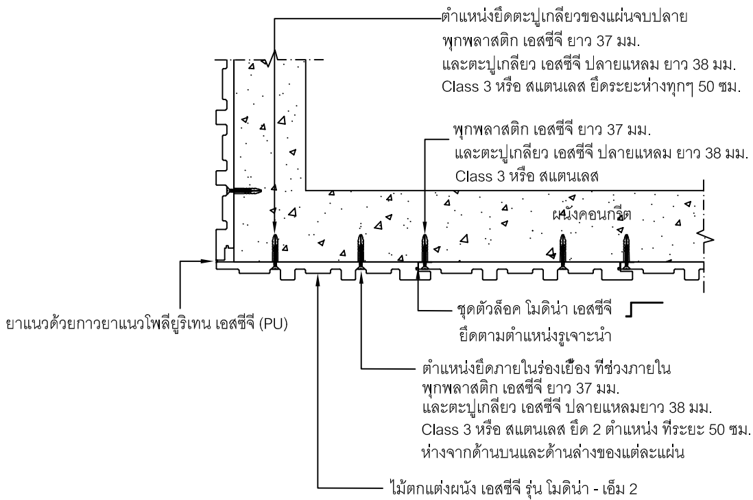
Detail จบงานมูนนอก
